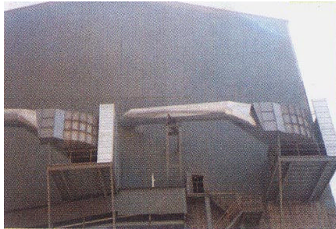
그림 1 항만 cement mill 토출기의 방음시설
